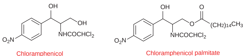
Fig. 7.15: Tasteless chloramphenicol palmitate.
