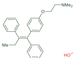
Tamoxifen
